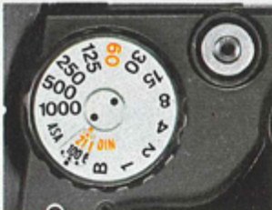
Zeiteinstellknopf: Gewünschte Verschlusszeiten können Sie durch Drehen am Verschlusszeitenknopf einstellen.
